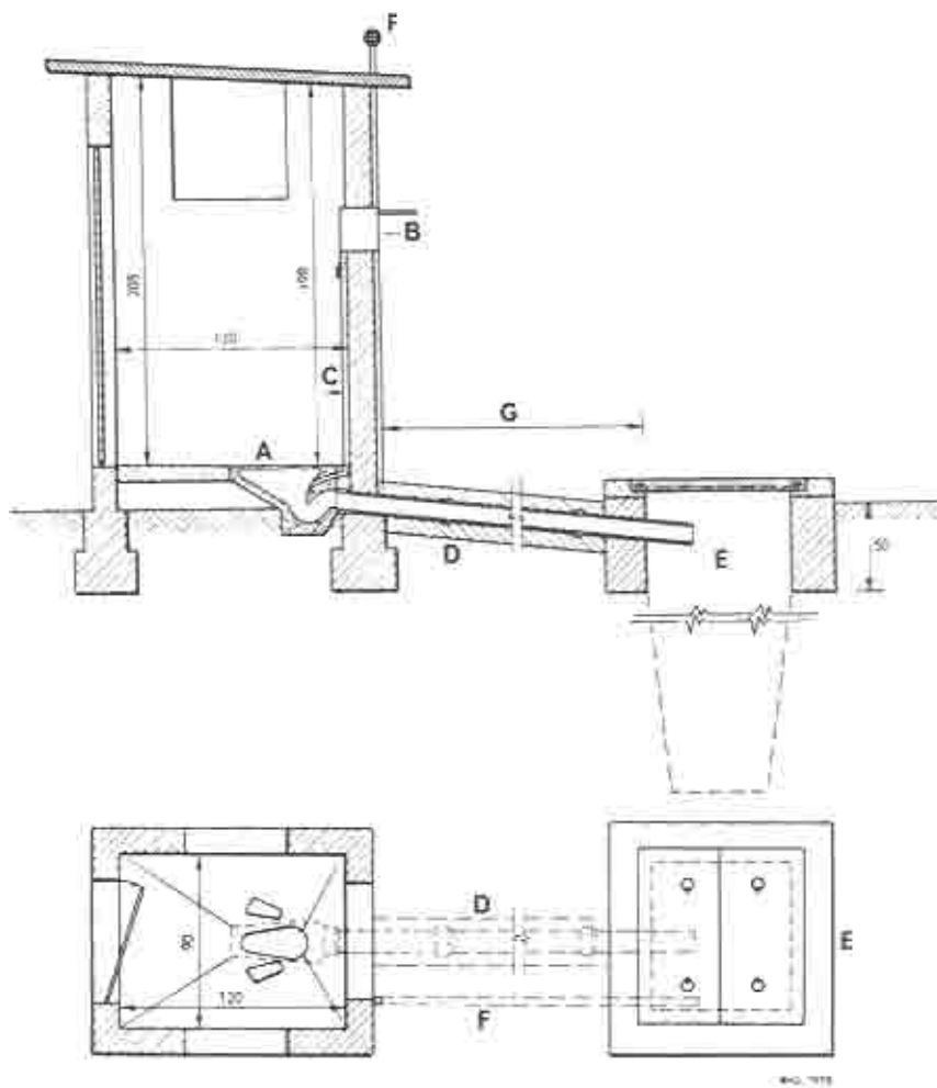
Fig. 34. POUR-FLUSH WATER-SEAL LATRINE
