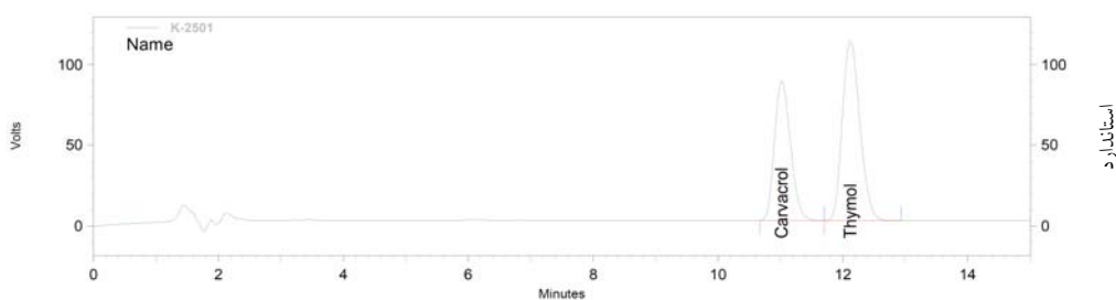
شکل شماره ۱- کروماتوگرام تیمول و کارواکربول در نمونه استاندارد و ۱۰۰ میلی‌مولار با دستگاه HPLC
