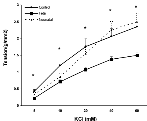
نمودار ۱- تانسیون حاصل از غلظت‌های مختلف کلرورپتاسیم بر بافت آئورت
